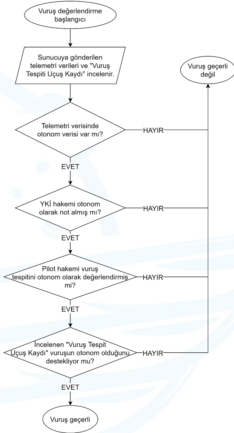
Şekil 2: Vuruş Tespiti Akış Şeması
